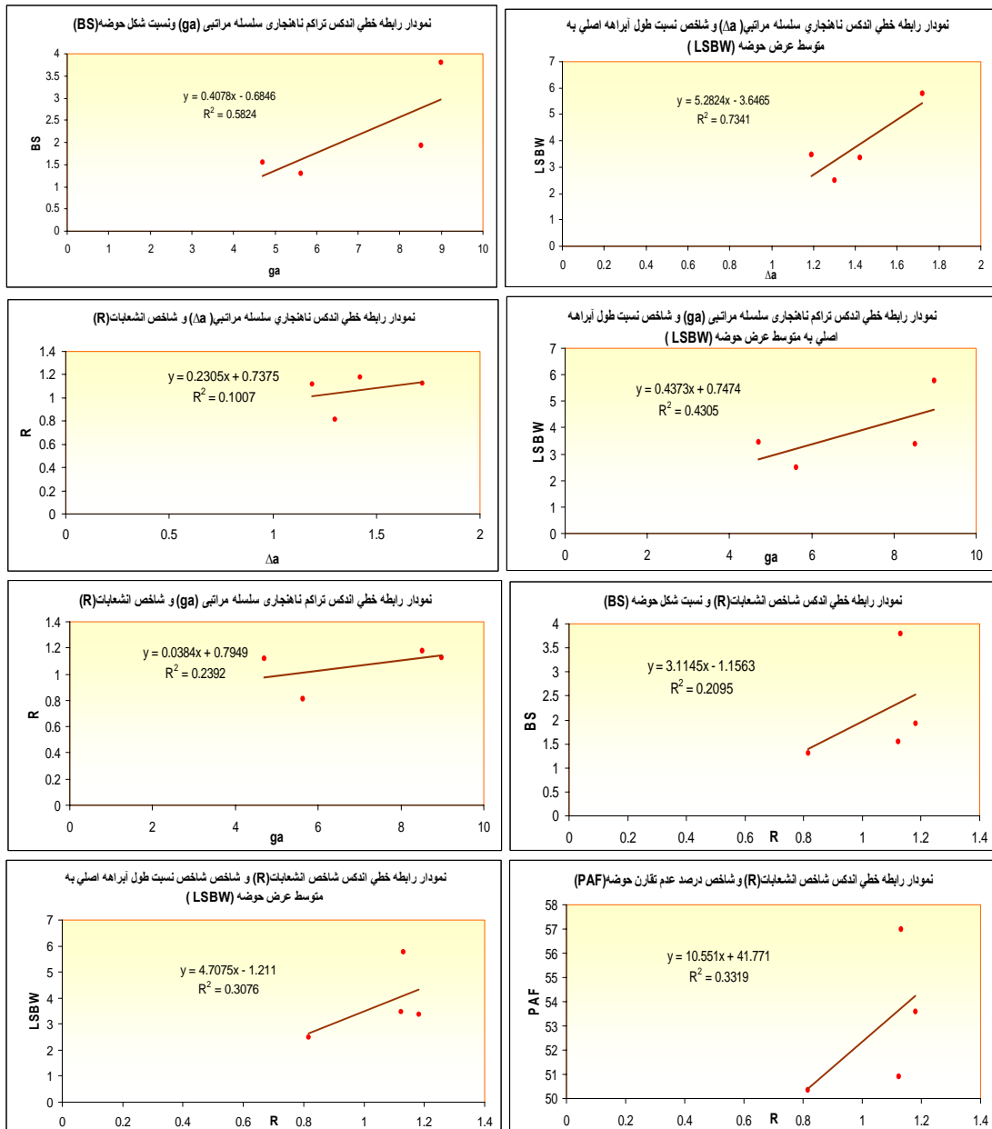
شکل ۴: رابطه خطی و مقدار ضریب تبیین بین \Delta a ، ga و R و پارامترهای BS ، PAF ، LSBW در حوضه‌های مورد مطالعه (منبع: نگارندگان)
